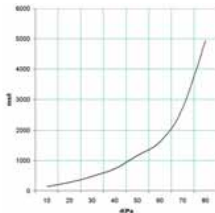
Evakuierungszeit (ms/l=s/m³) bei verschiedenen Vakuumgraden (-Kpa)
