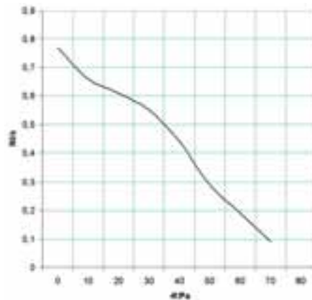
Luftmenge (NI/s) bei verschiedenen Vakuumgraden (-Kpa)
