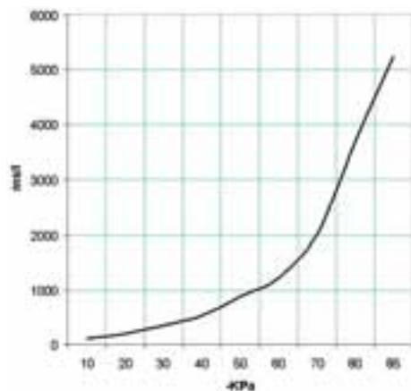
Evakuierungszeit (ms/l=s/m³) bei verschiedenen Vakuumgraden (-Kpa)
