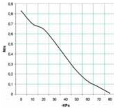
Luftmenge (NI/s) bei verschiedenen Vakuumgraden (-KPa)
