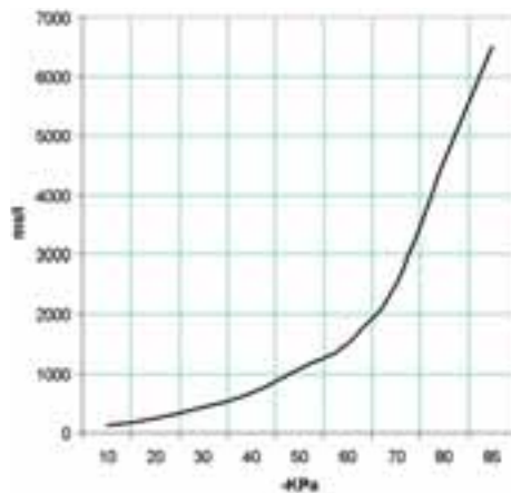
Evakuierungszeit (ms/l = s/m 3 ) bei verschiedenen Vakuumgraden (-KPa)
