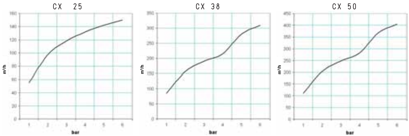
Menge der ausgeblasenen Luft (m 3 /h) bei verschiedenen Werten des Versorgungsdrucks (bar)
