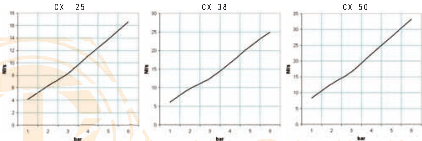
Luftverbrauch (l/s) bei verschiedenen Werten des Versorgungsdrucks (bar)
