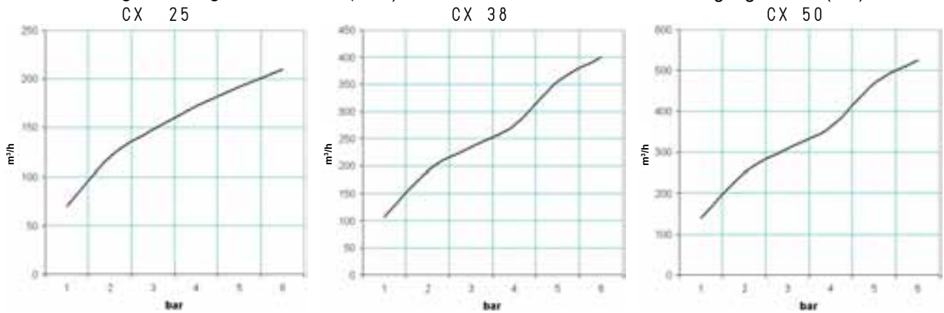
Vakuumgrad (-Kpa) bei verschiedenen Werten des Versorgungsdrucks (bar)
