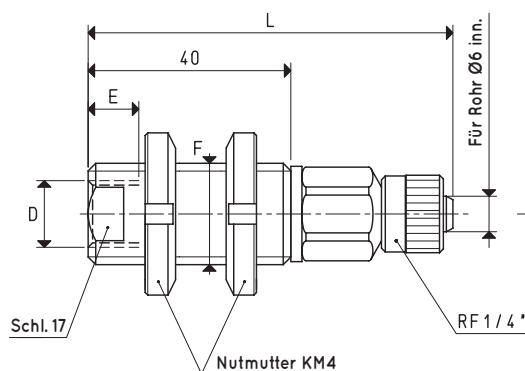
AUSFÜHRUNG 02 91 01
