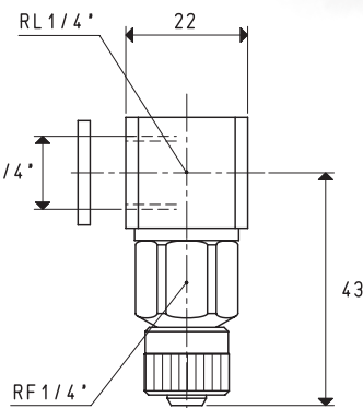
AUSFÜHRUNG 02 91 01 L
