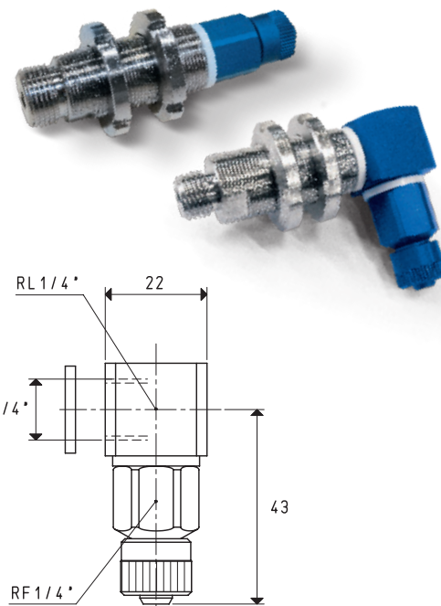
AUSFÜHRUNG 02 91 . . L
