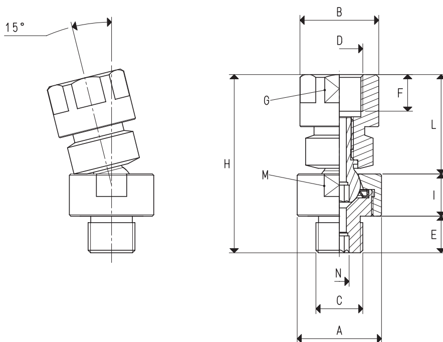
KUGELGELENKE MIT AXIALEM VAKUUMANSCHLUSS
