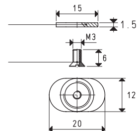
Befestigungsplatte Art. 00 08 97
